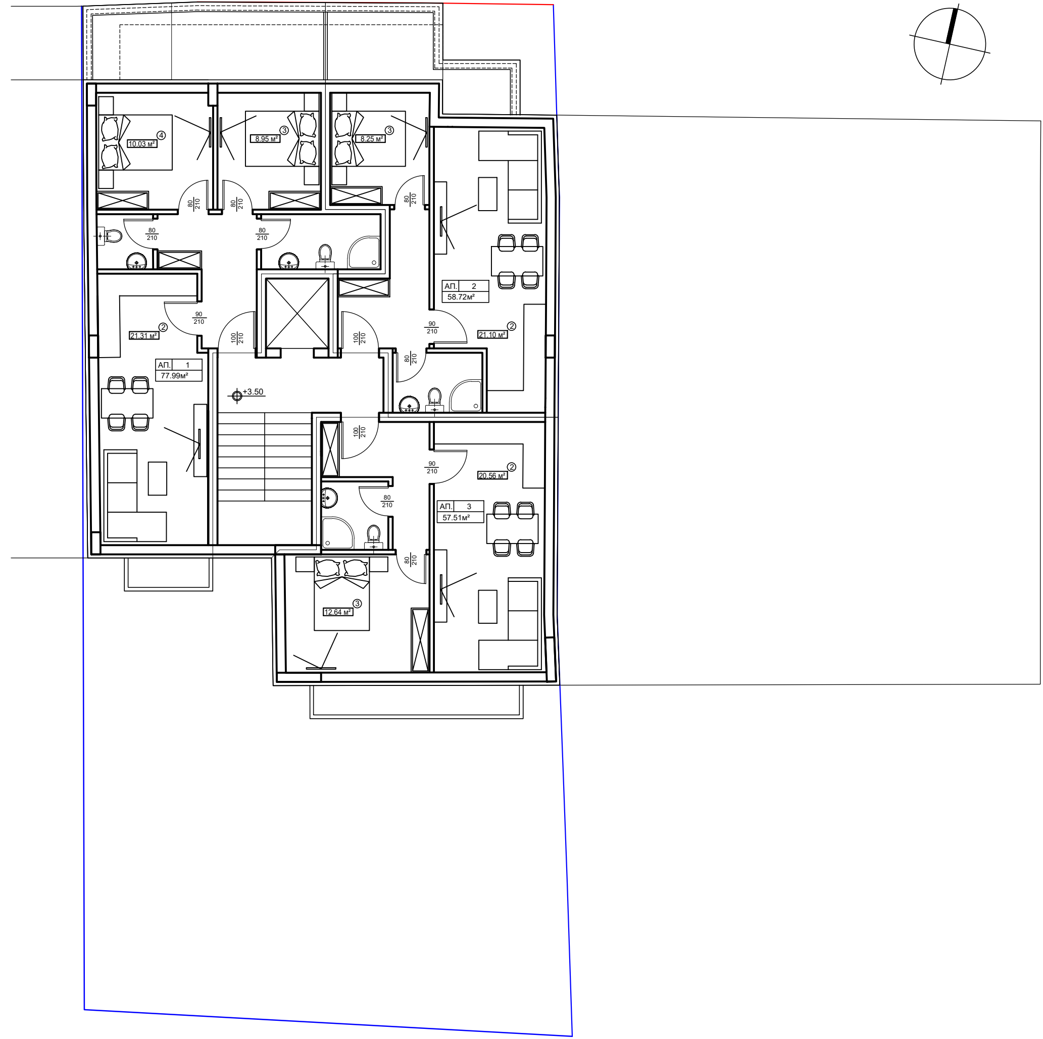
РАЗПРЕДЕЛЕНИЕ ВТОРИ ЕТАЖ 217,32м2
