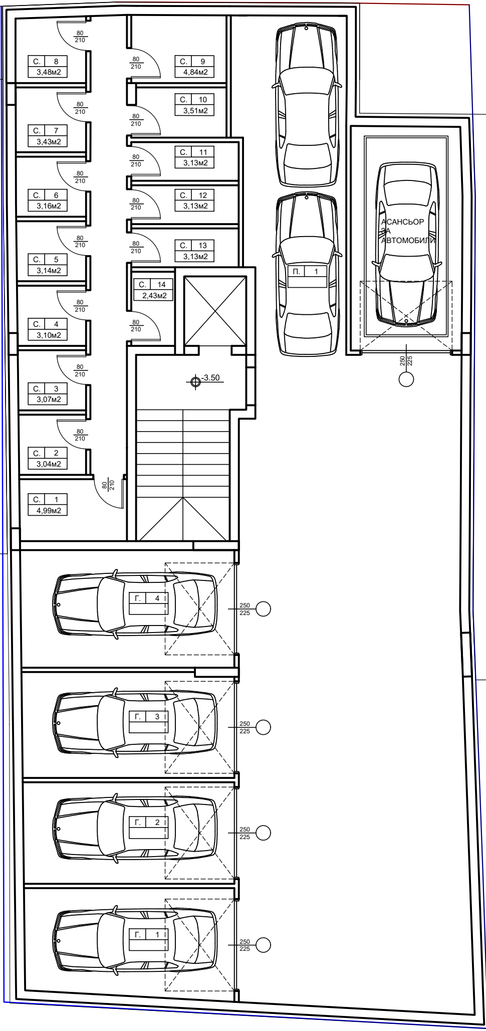
РАЗПРЕДЕЛЕНИЕ СУТЕРЕНЕН ЕТАЖ 348,48m 2
